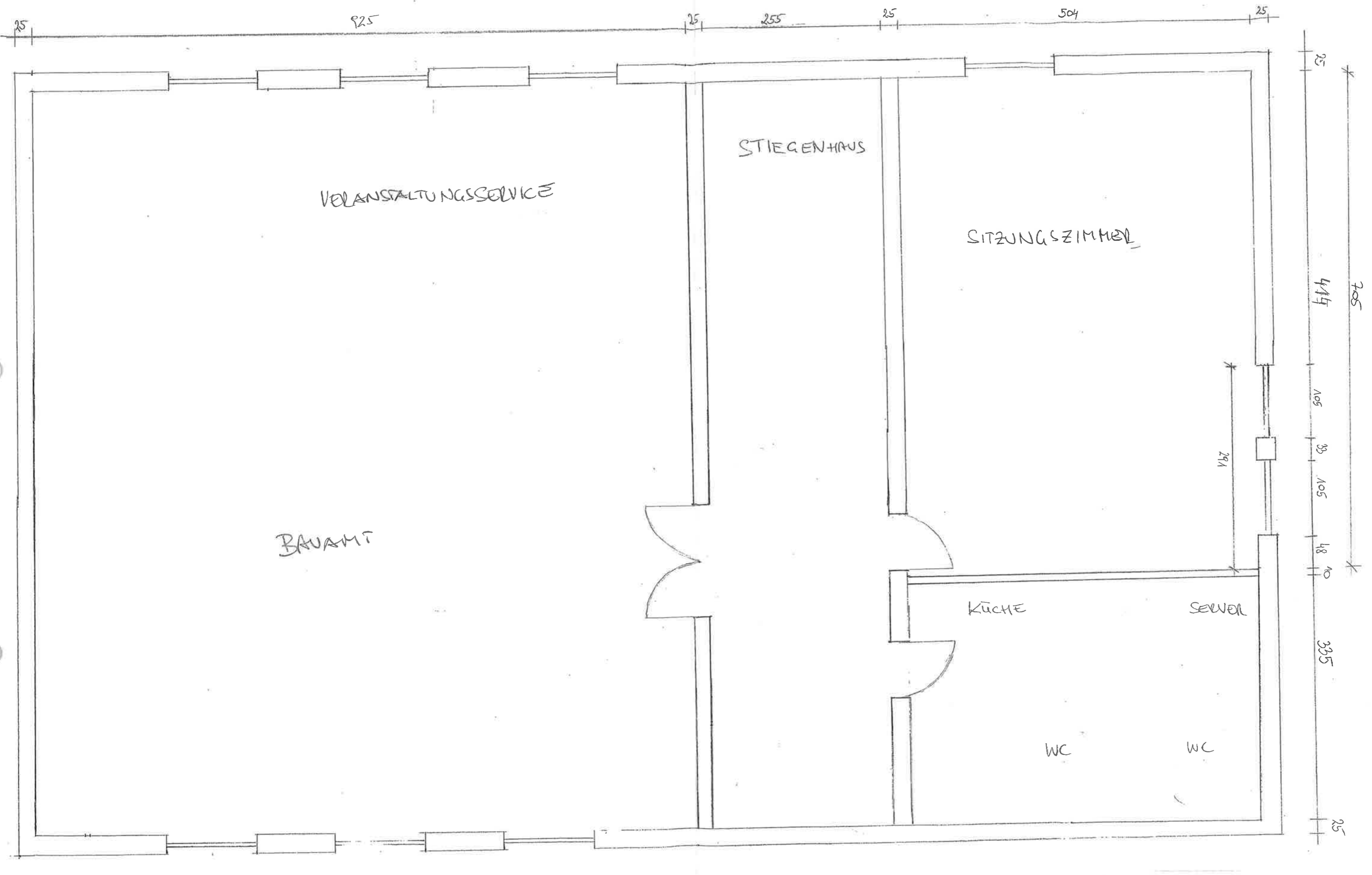
GRUNDRISS GEMEINDEAMT OBERGESCHOSS
