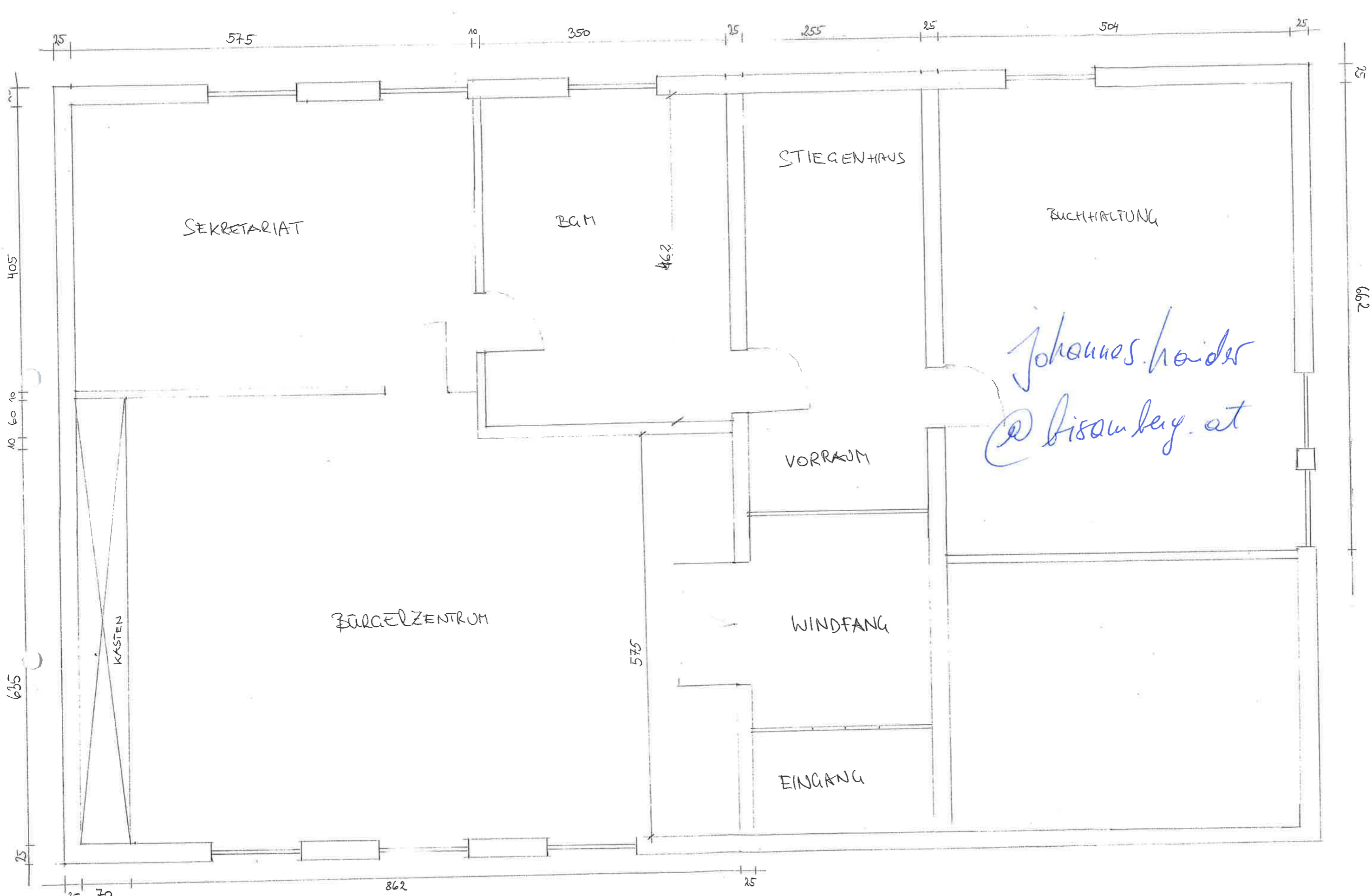
GRUNDRISS GEMEINDEAMT ERDGESCHOSS
